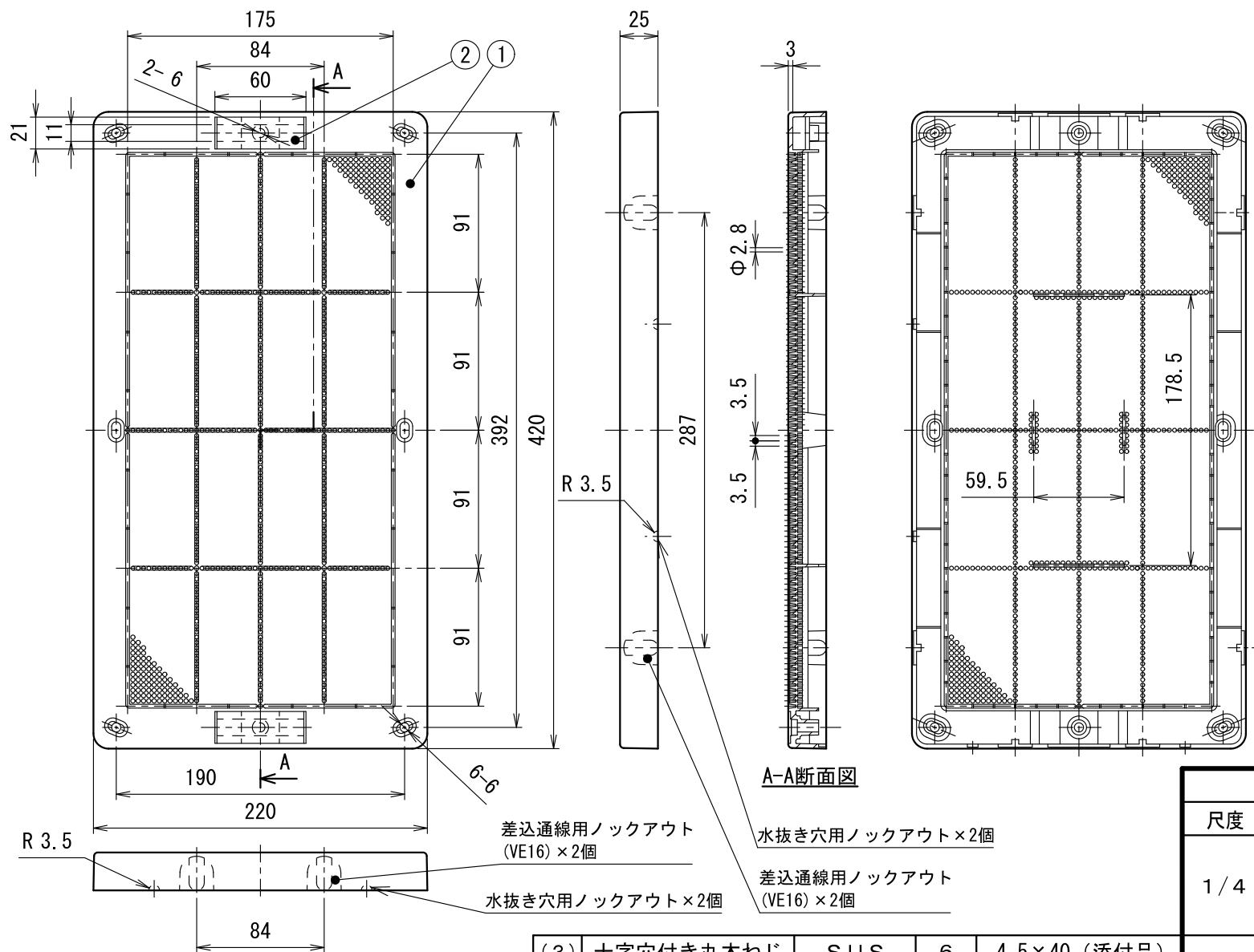
製品仕様図
